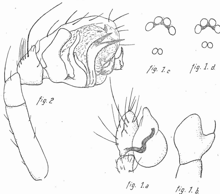
Fig. 1 - Paraleptoneta franciscolori sp. n. a ♂ palpi tarsus et latere visus, b ♂ palpi tibia desuper visa, c Oculi exemplaris typici, d Oculi exemplaris caveae «dell'Acqua».
